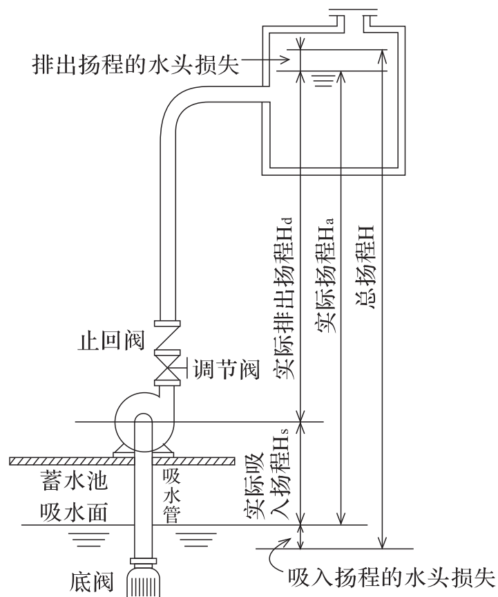
泵的提水系统
