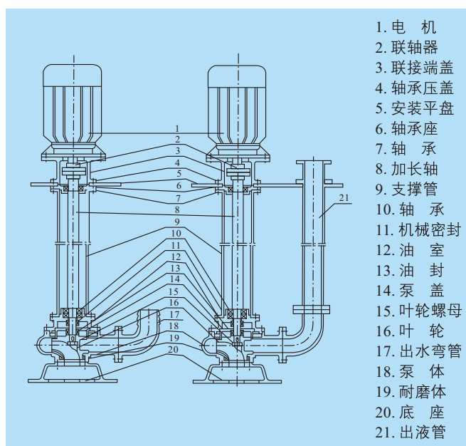
YW 型泵结构示意图
