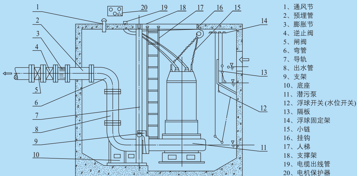
固定式安装示意图
