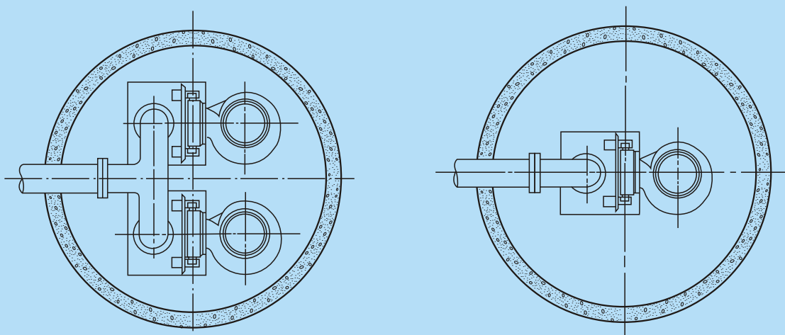
双导轨双泵排水平面图
