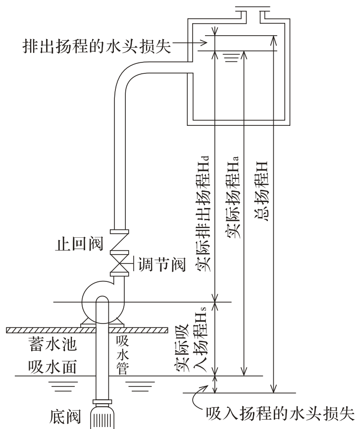
泵的提水系统
